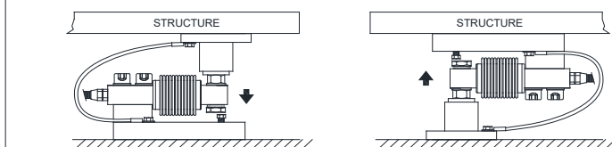
FIJACIÓN A LA ESTRUCTURA PESADA
